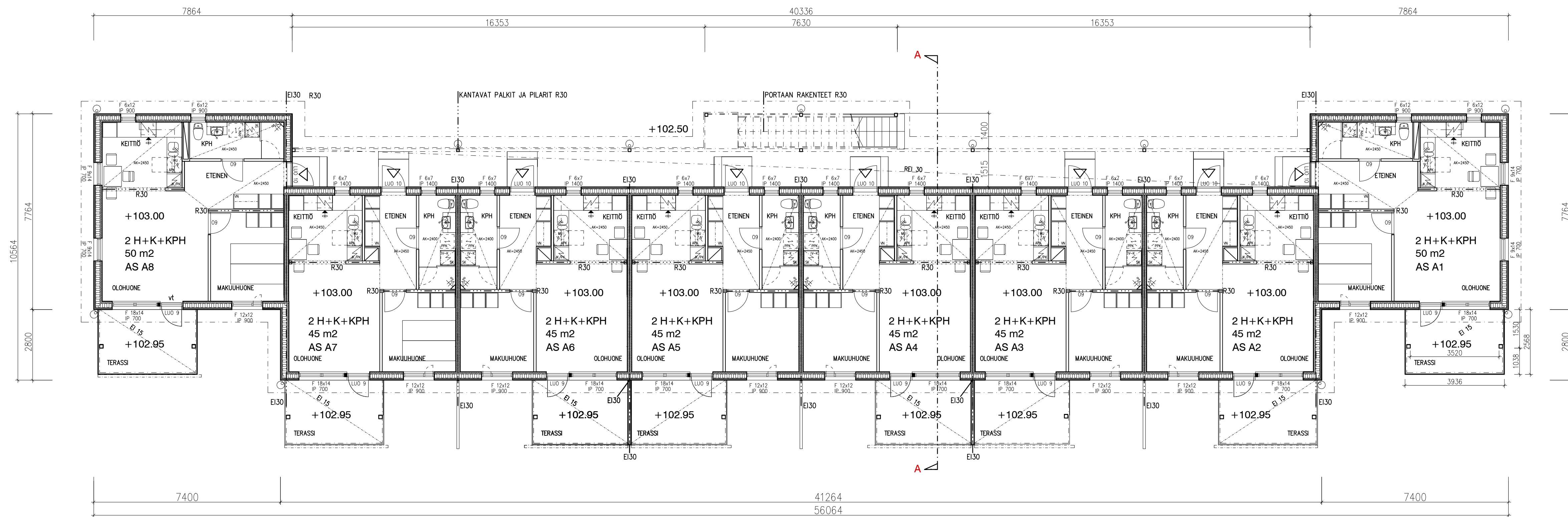
RAKENNUS A 1. KERROS POHJA 1 : 100
