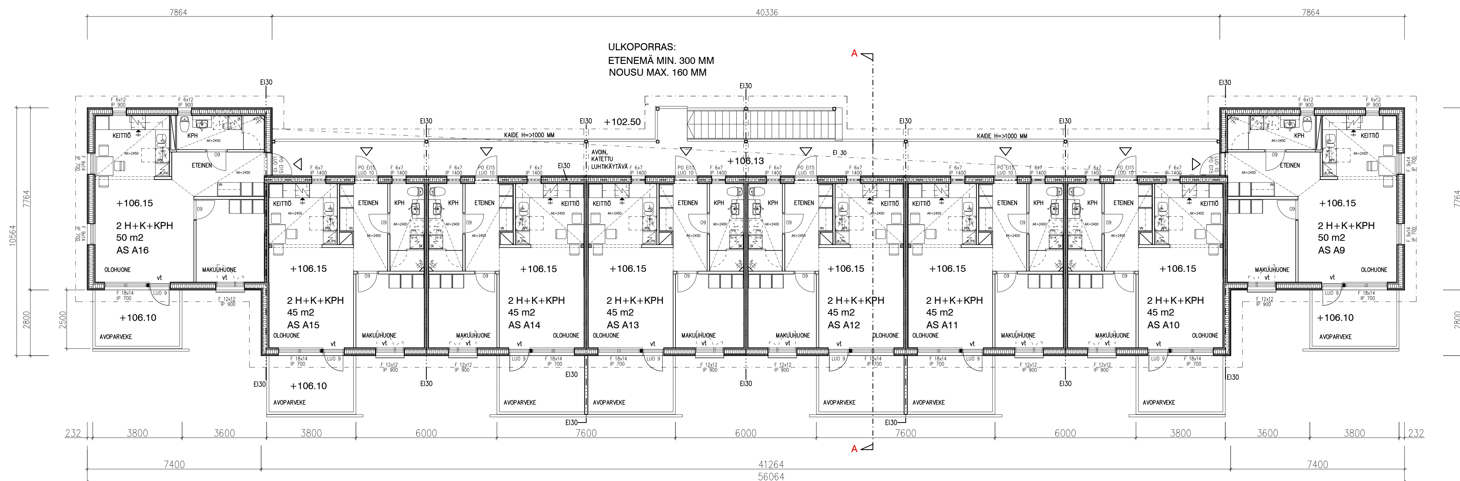
RAKENNUS A 2. KERROS POHJA 1 : 100
